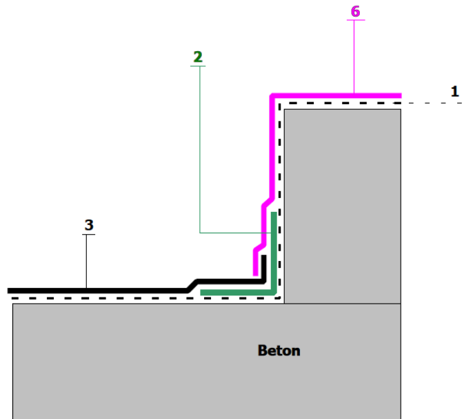
Fig. 4 – Detail opstand
