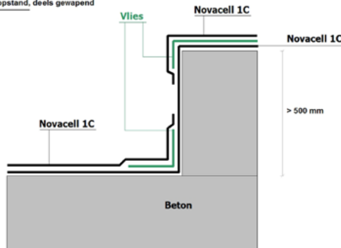
Detail opstand, deels gewapend
