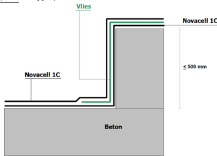
Detail opstand, volledig gewapend
